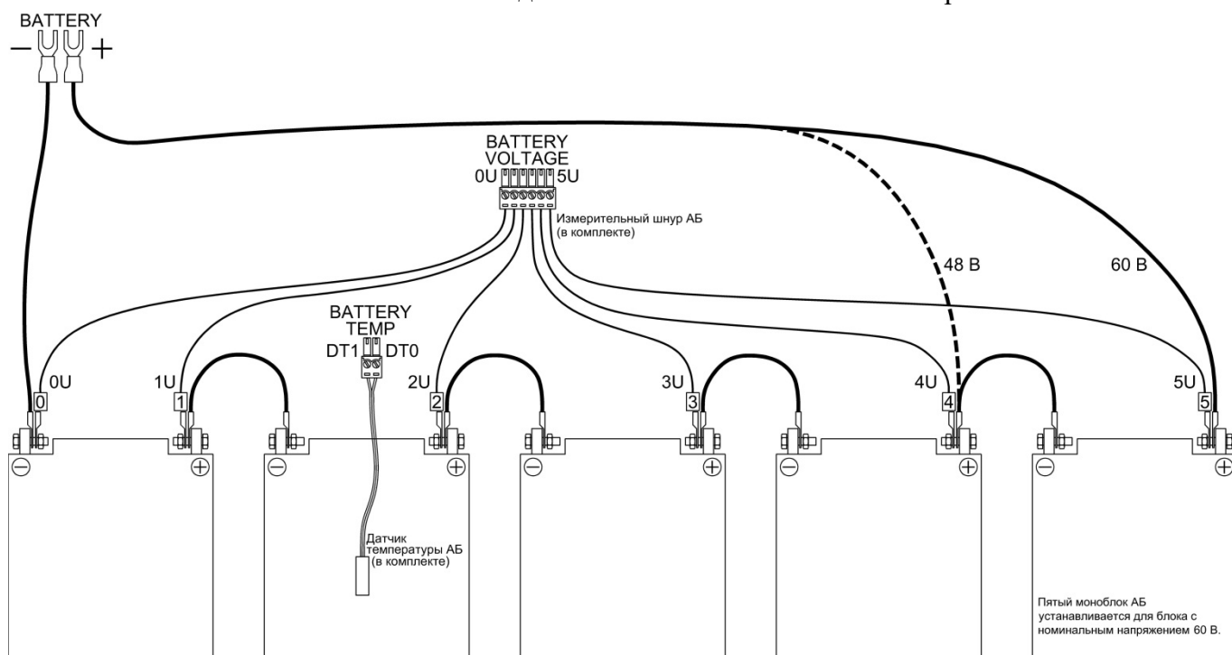
Рис. 8. Подключение АБ.
