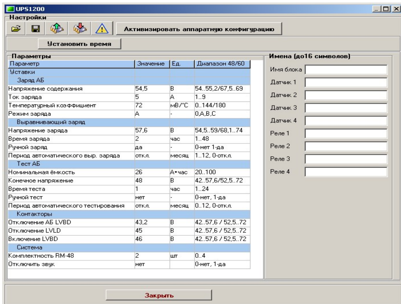
Рис. 11. Основное окно программы. Авария 220 В, разряд АБ.
