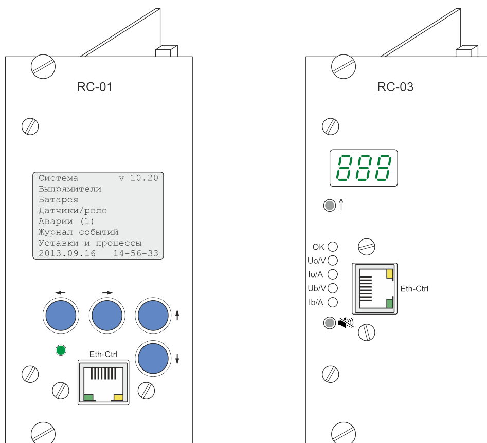
Рис.6. Вид лицевой панели модулей RC–01 и RC–03.
