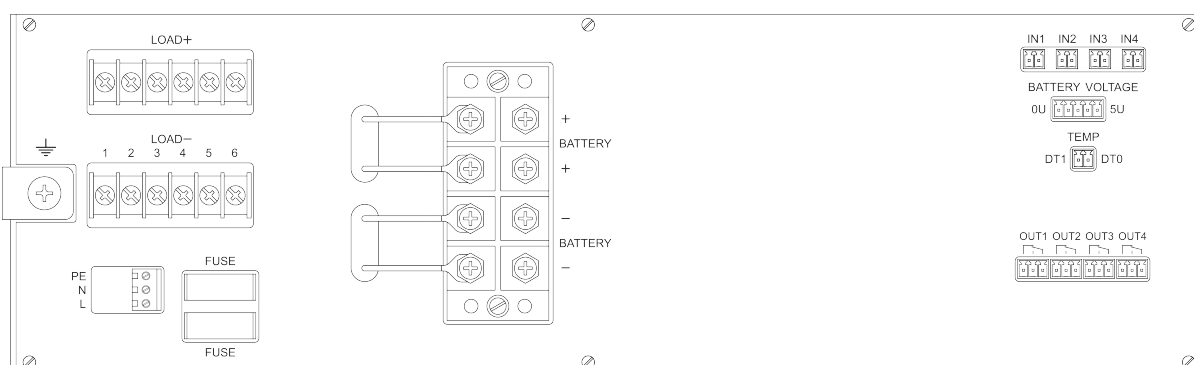
Рис.2. Задняя сторона блока MC04-UPS-48/60-1200.
