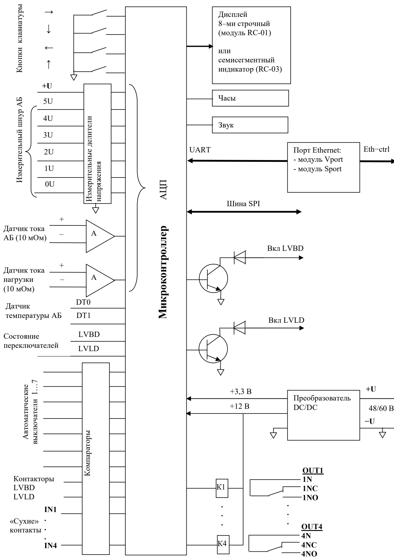
Рис.7. Функциональная схема модуля управления.
