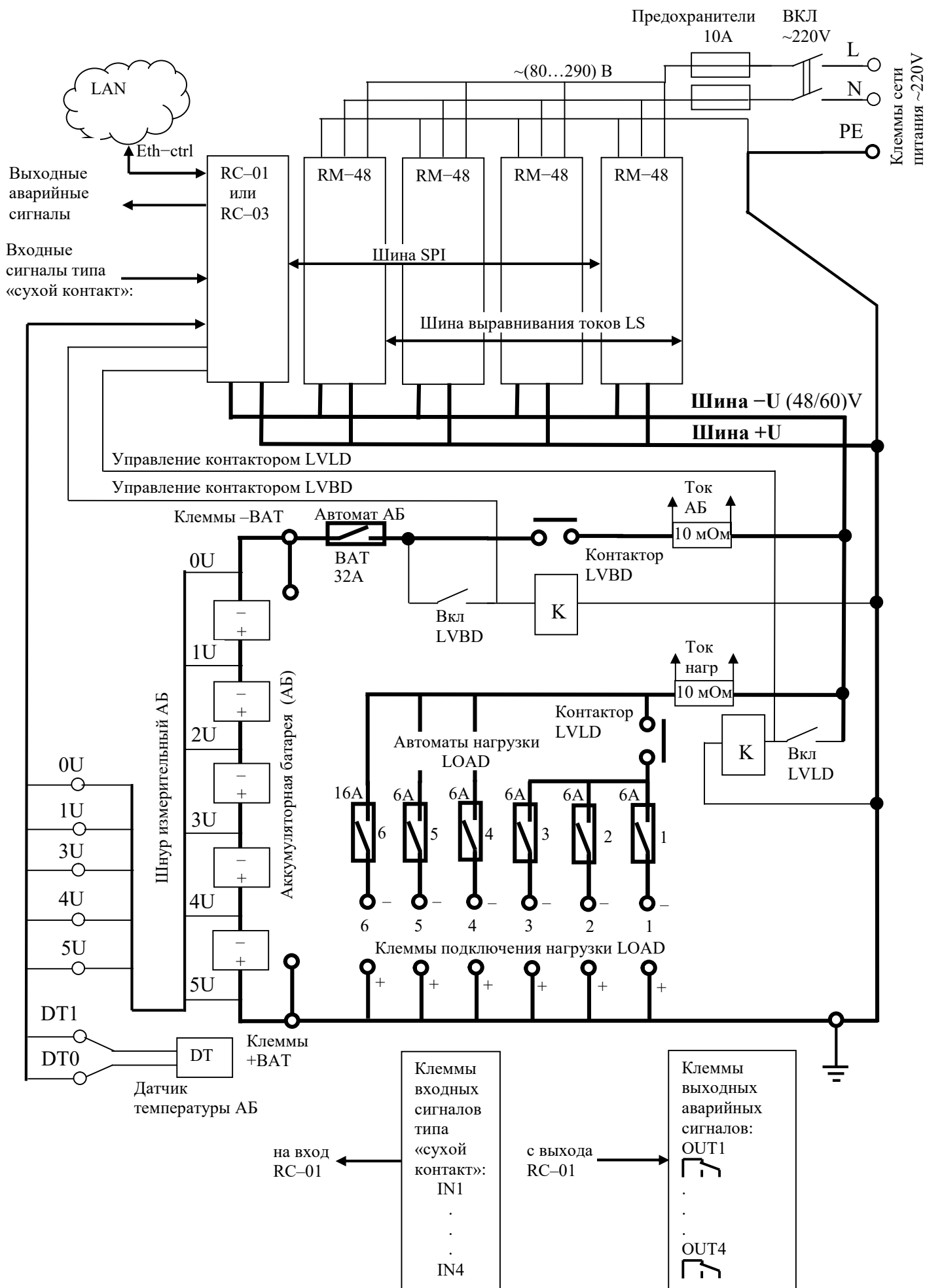
Рис. 3. Функциональная схема блока MC04-UPS-48/60-1200.
