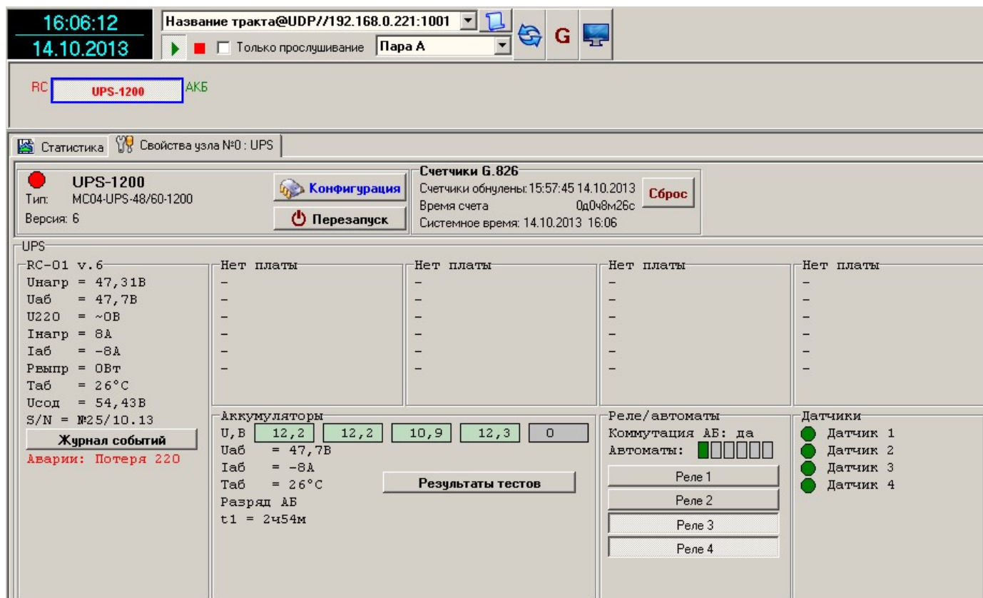
Рис. 12. Окно конфигурации. Задание уставок параметров и управление процессами.
