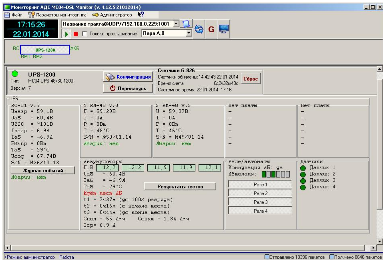
Рис. 10. Основное окно программы. Режим теста АБ.
