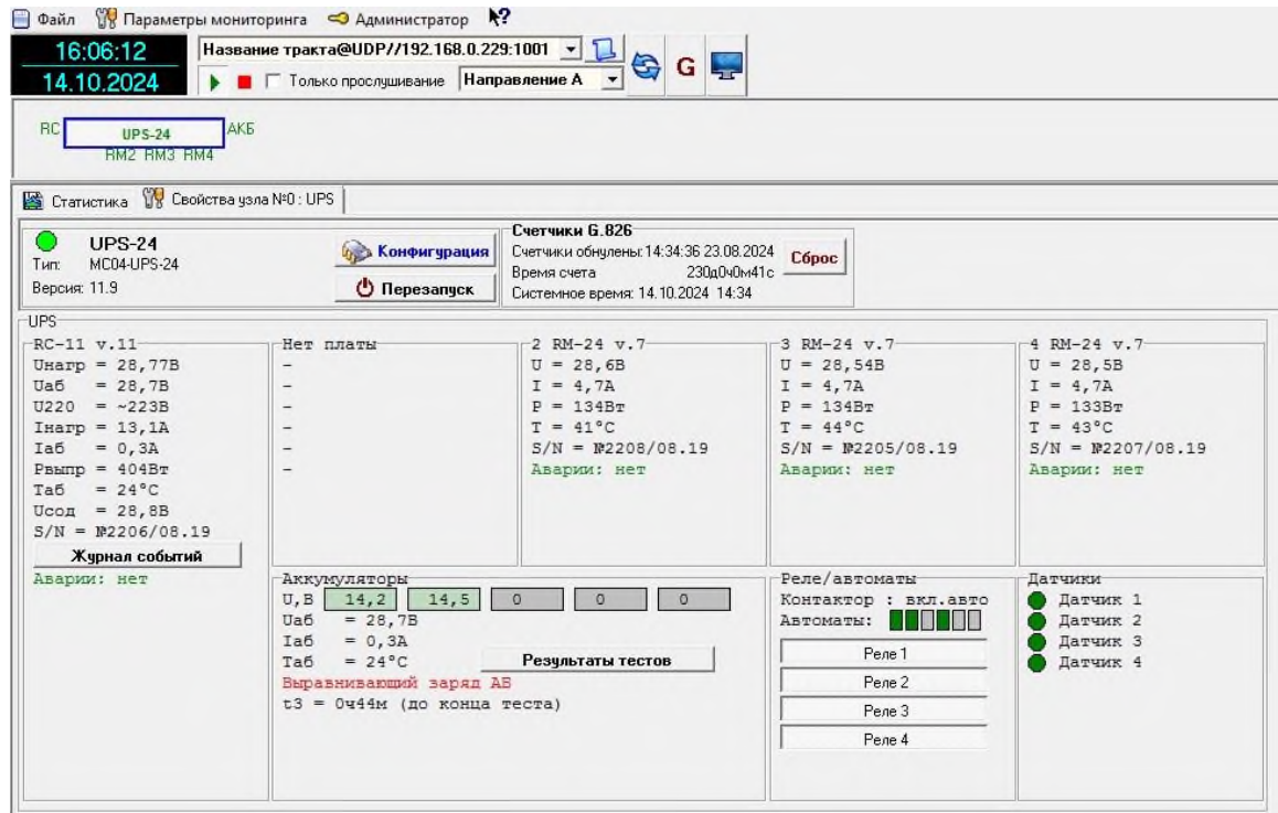
Рис. 10. Основное окно программы. Выравнивающий заряд АКБ.
