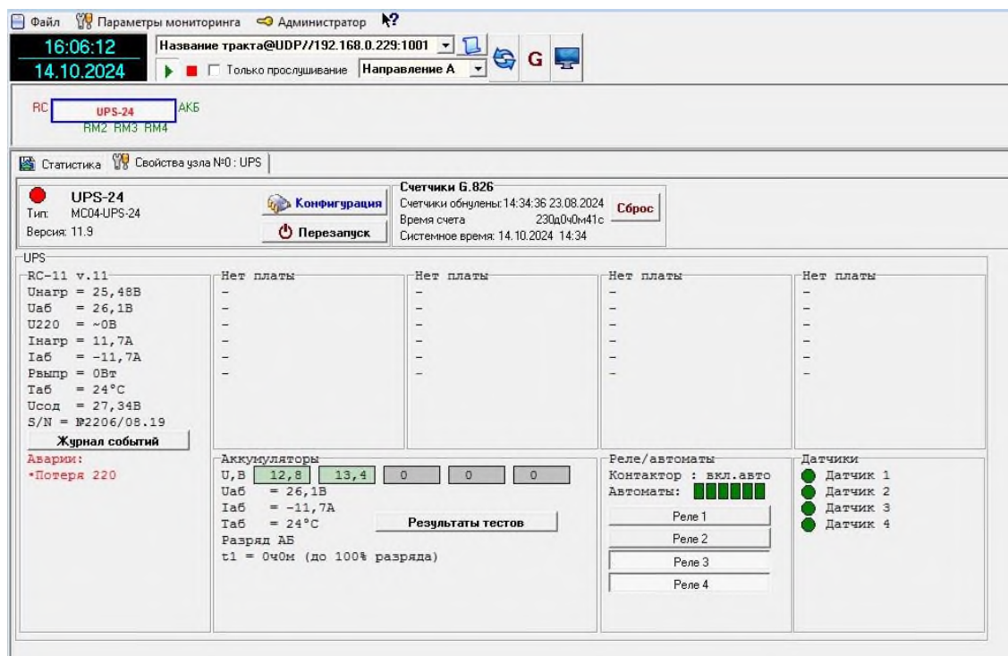
Рис. 11. Основное окно программы. Авария 220 В, разряд АКБ.
