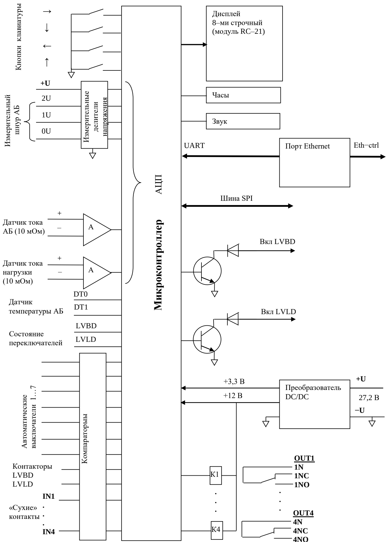
Рис.6. Функциональная схема модуля управления RC-21.
