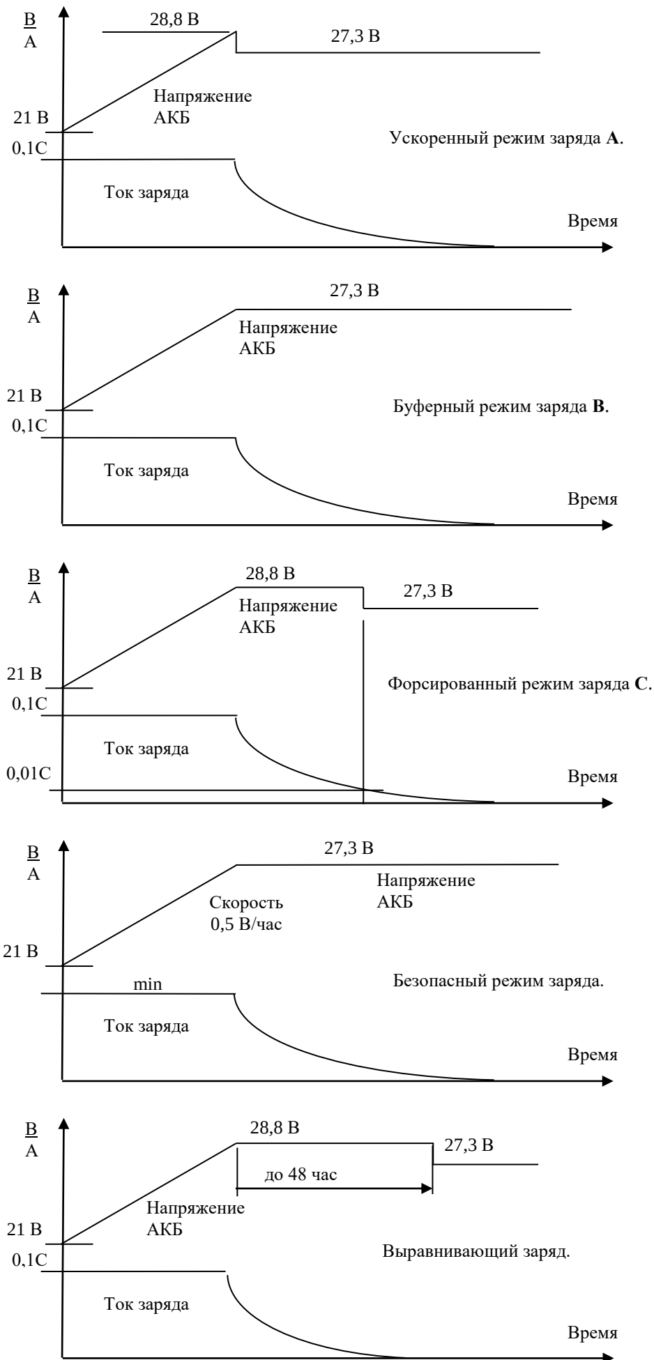
Рис. 4. Режимы заряда АКБ.
