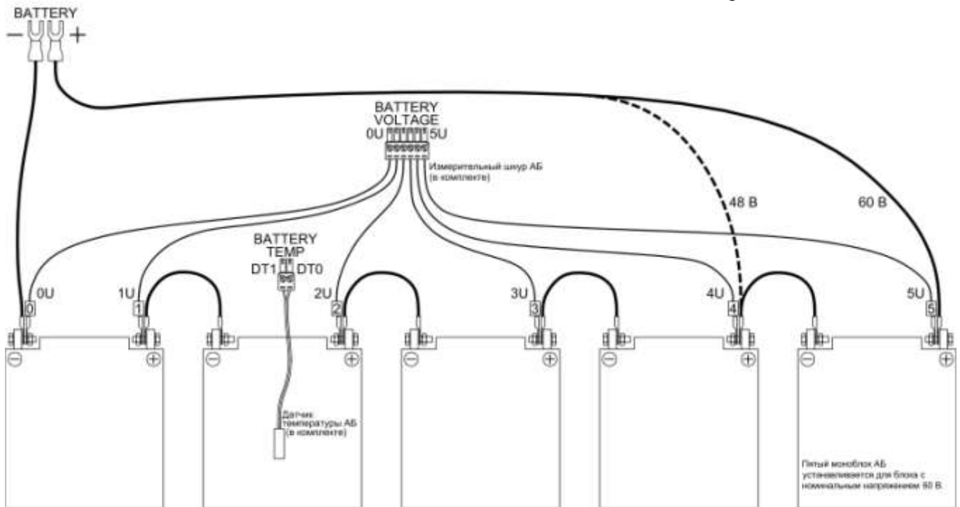
Рис. 7. Подключение АБ.
