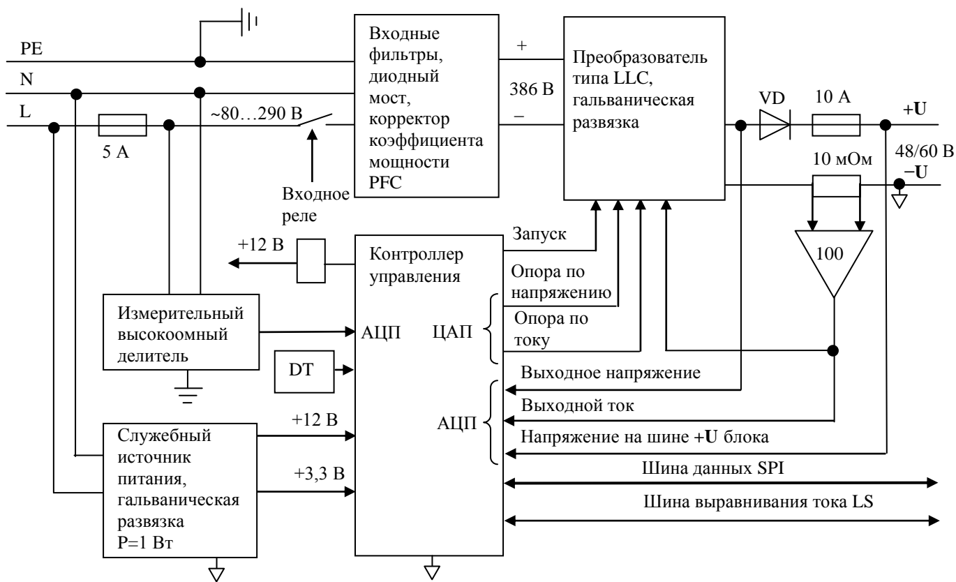
Рис. 5. Функциональная схема выпрямителя RM–48.
