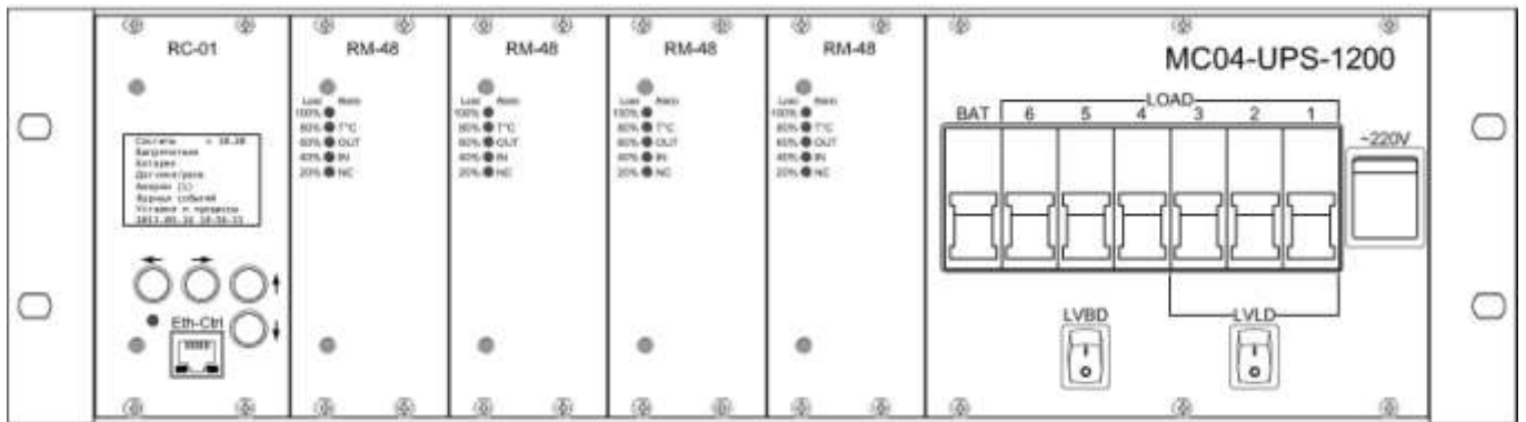
Рис.1. Лицевая сторона блока MC04–UPS–1200.
