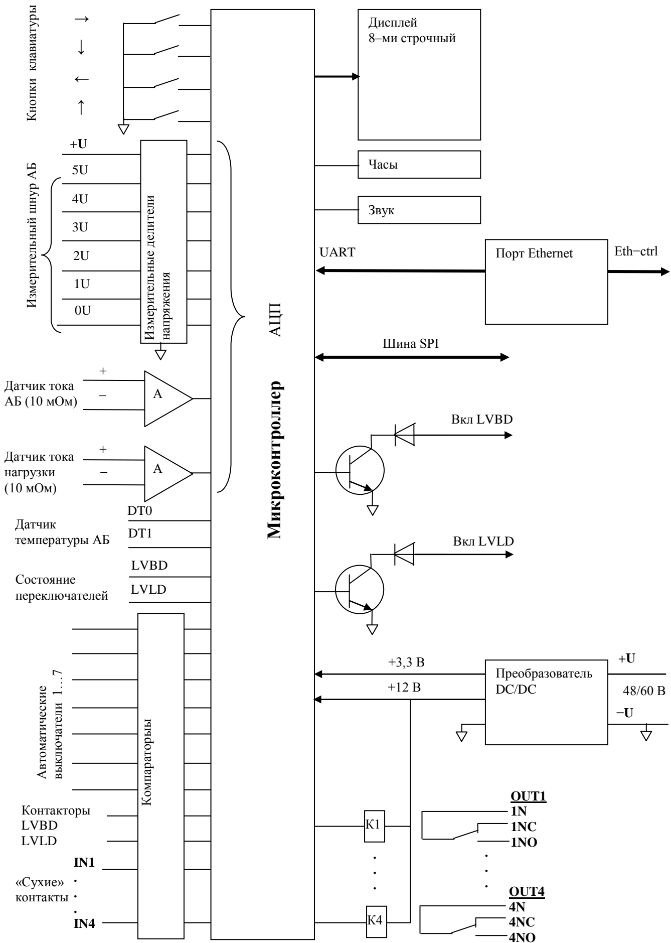
Рис.6. Функциональная схема модуля управления RC-01.
