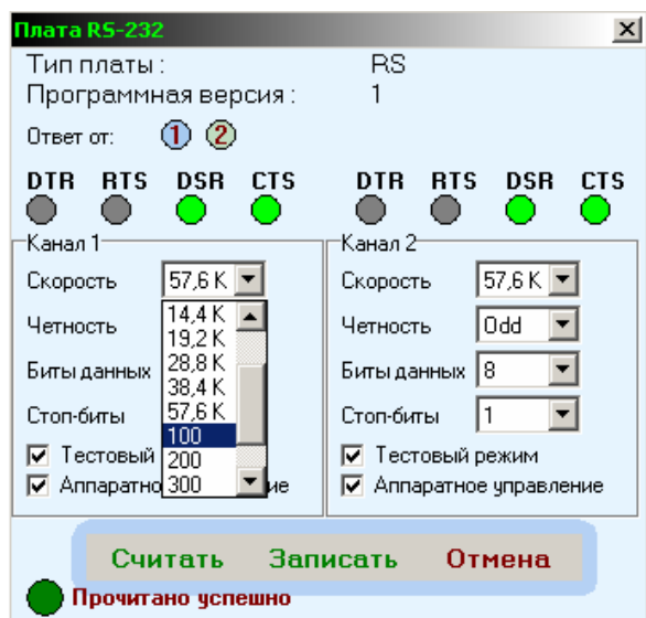
Рис.3. Окно конфигурации платы RS-232.
