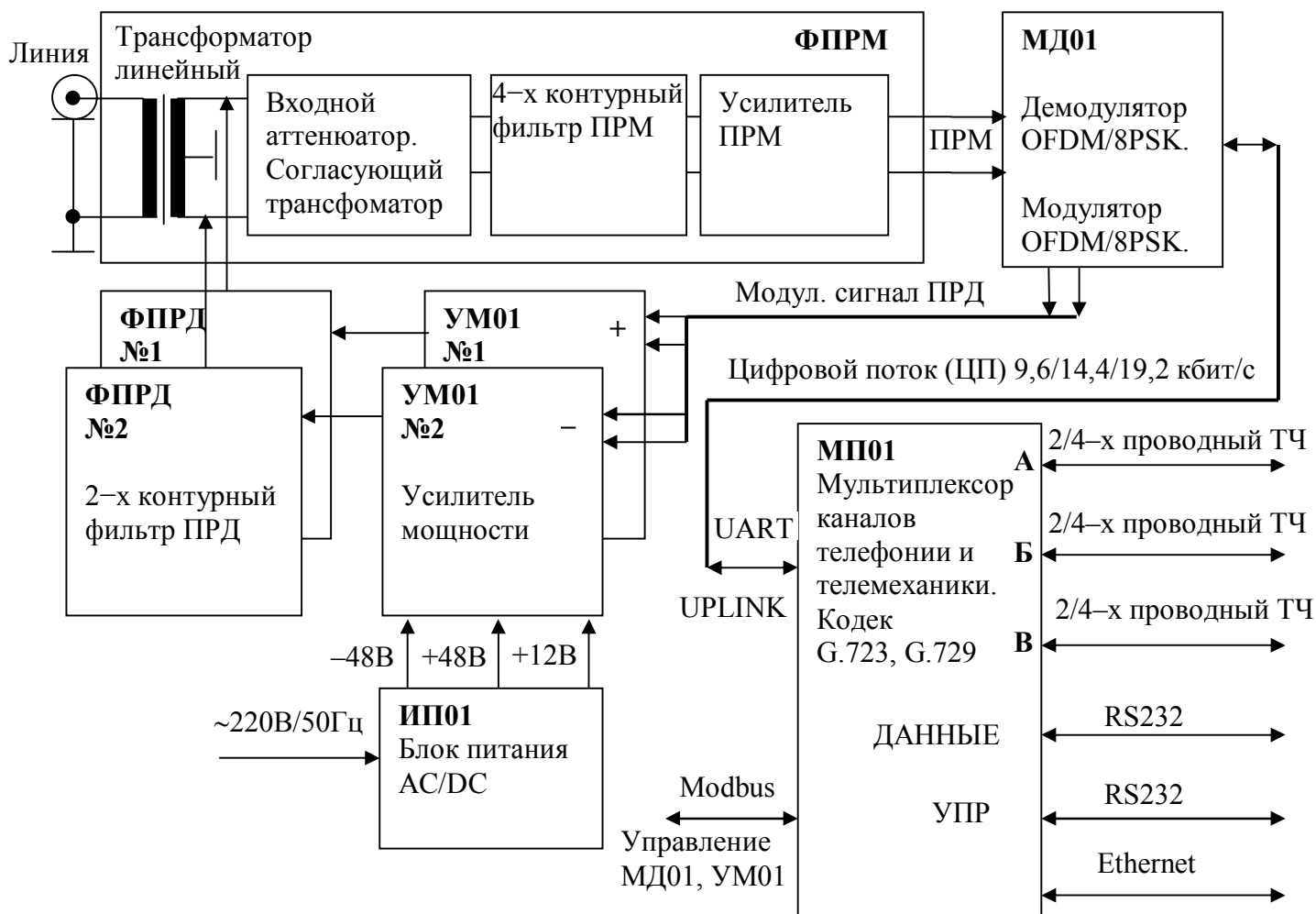
Рис.1. Структурная схема блока MC04-PLC.
