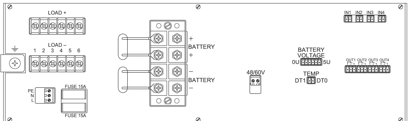
Рис.2. Задняя сторона блока MC04-UPS-1200.
