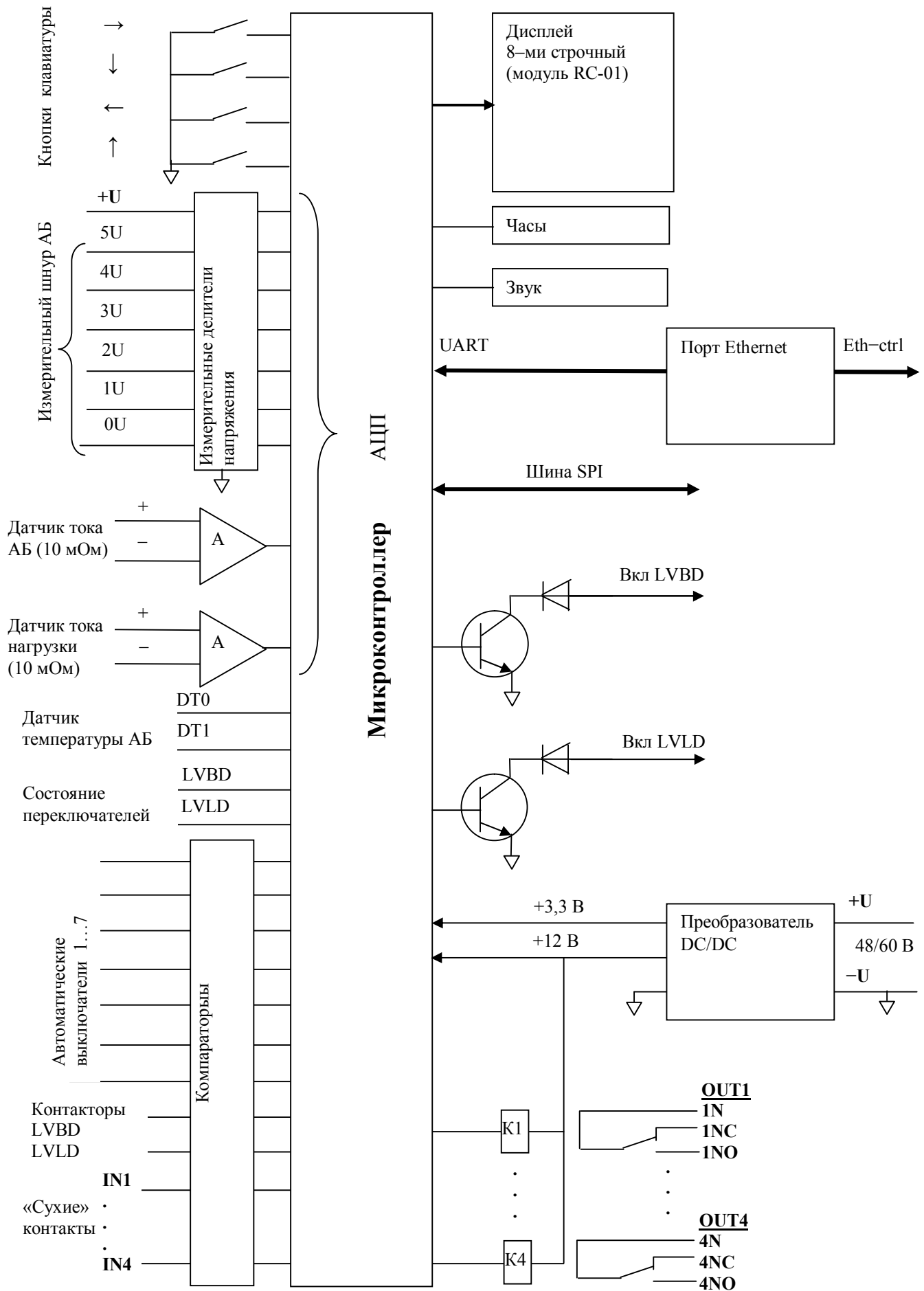
Рис.6. Функциональная схема модуля управления RC-01(RC-02).
