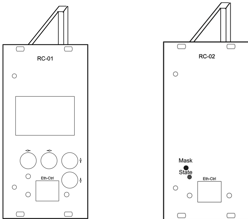
Рис.6. Вид лицевой панели модулей RC-01 и RC-02.
