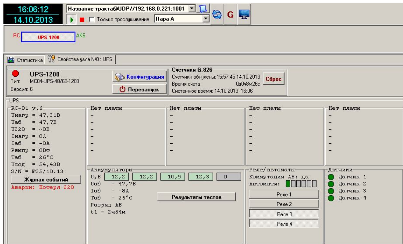
Рис. 11. Основное окно программы. Авария 220 В, разряд АБ.
