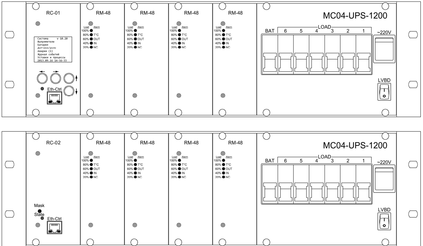
Рис.1. Лицевая сторона блока MC04-UPS-1200 с платой RC-01 и с платой RC-02.
