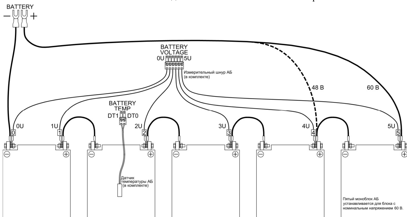
Рис. 7. Подключение АБ.
