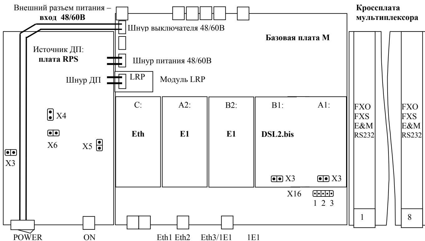
Рис. 5а. Схема расположения узлов модем-мультиплексора MC04-DSL2.bis-xxx-RPS.
