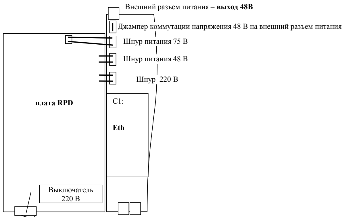
Рис. 4б. Схема расположения узлов модем-мультиплексора MC04-DSL.F-xxx-220V.
