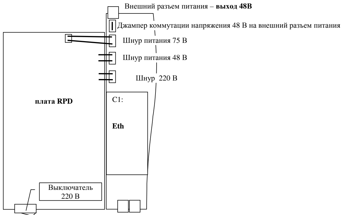
Рис. 46. Схема расположения узлов модем-мультиплексора MC04-DSL.F-xxx-220V.
