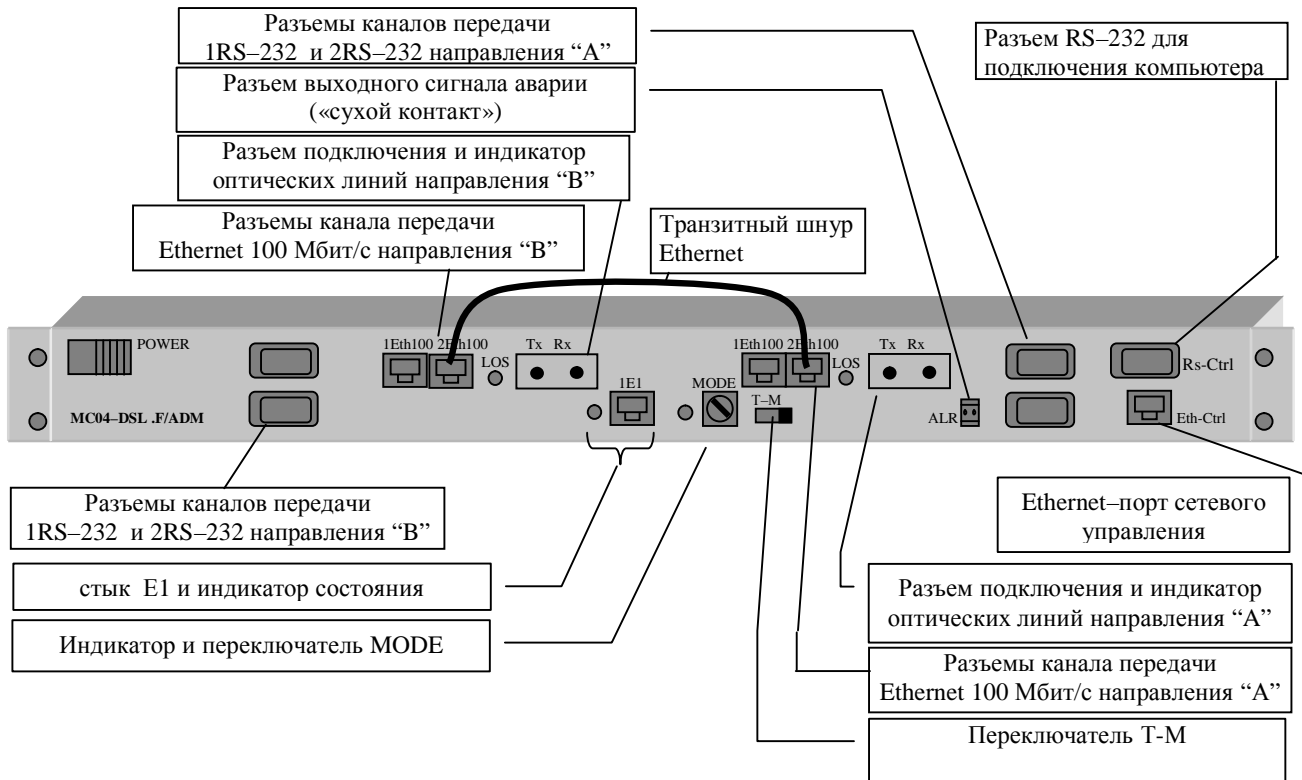
Рис. 1. Модем в корпусе 1U.
