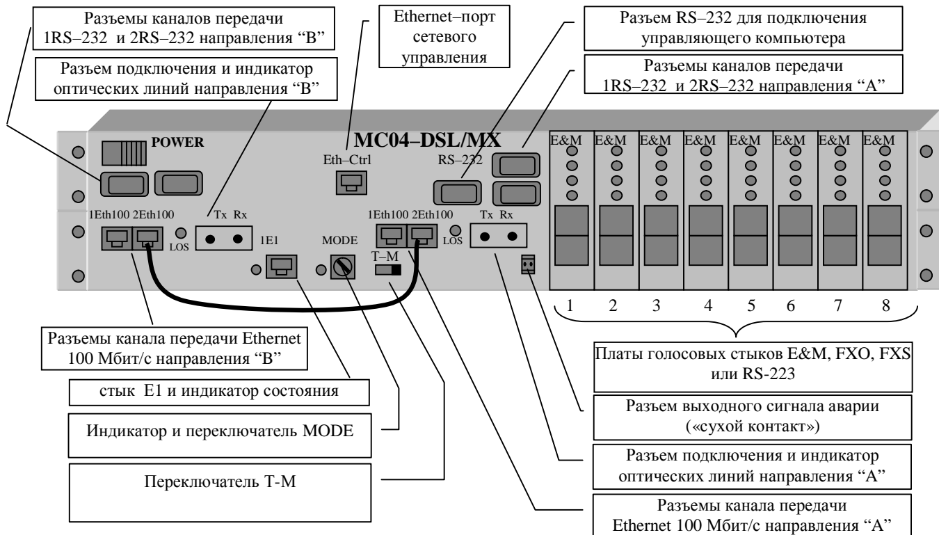
Рис. 2. Модем-мультиплексор на 8 плат канальных оконечий в корпусе 2U.
