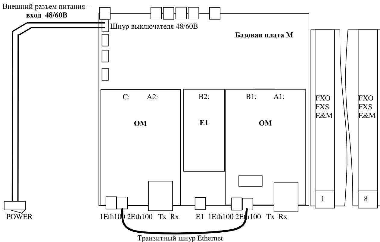
Рис. 4а. Схема расположения узлов модем-мультиплексора MC04-dsl.F-xxx- 60V.
