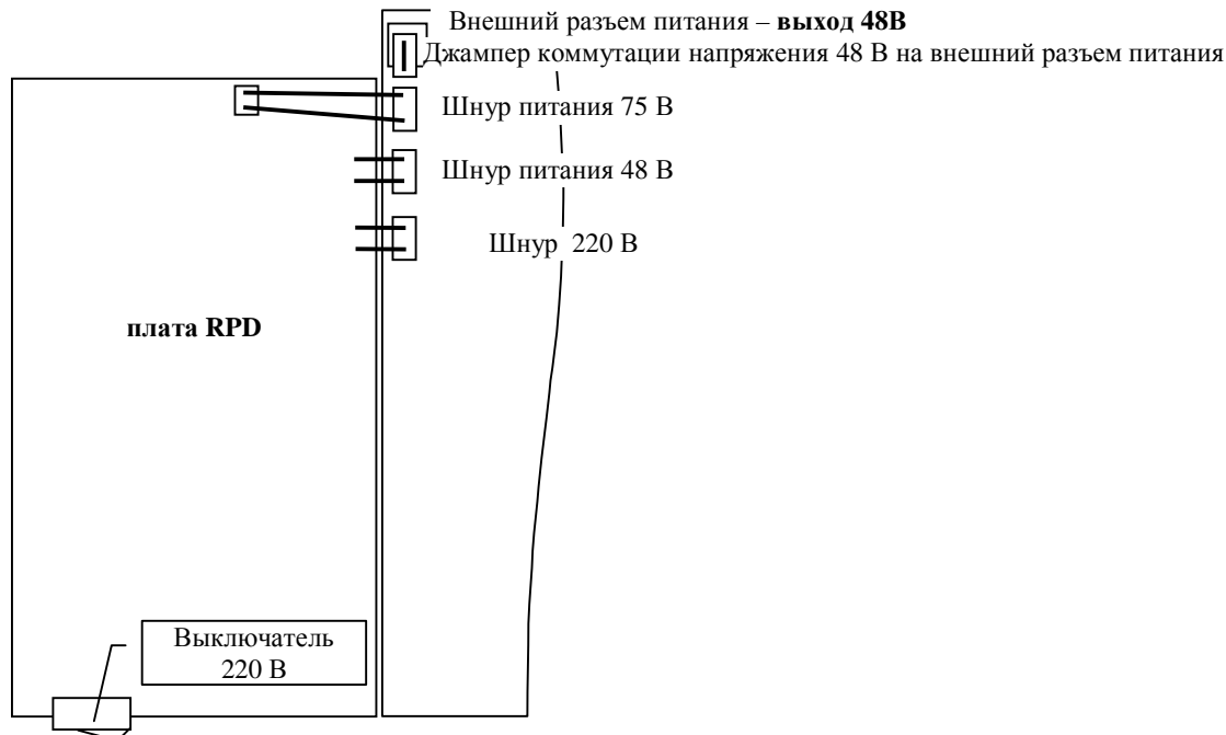
Рис. 4б. Схема расположения узлов модем-мультиплексора MC04-DSL.F-xxx-220V.
